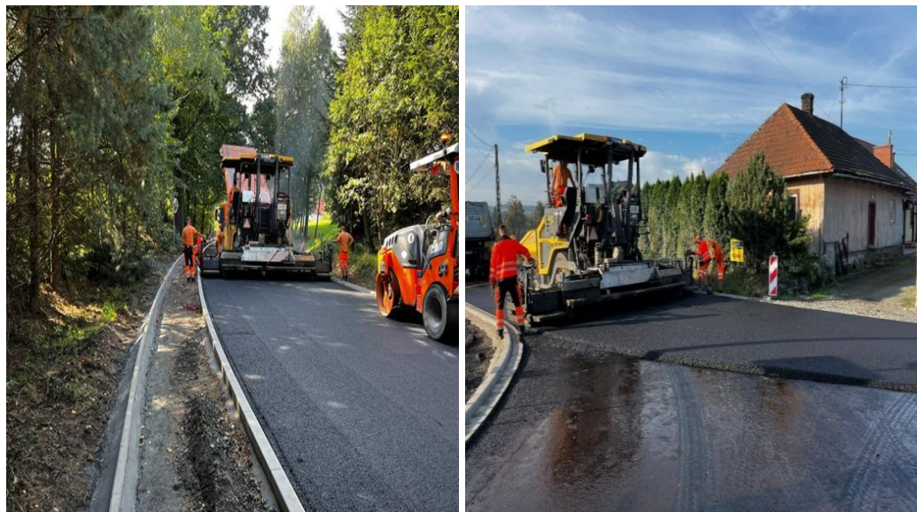
Fot. 47 Przebudowa drogi powiatowej nr 2071K w km od 15+380,00 do km 16+159,47 w miejscowościach Grabie i Lubomierz, Powiat Bocheński
